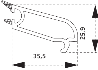
PVN1460BY Tek Cam Çıtası Single Glazing Bead
