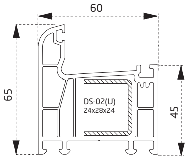
PRVNEC01B Kasa Profili Frame Profile
