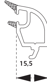
PVN1960BY 24 mm Cam Çıtası 24mm Glazing Bead
