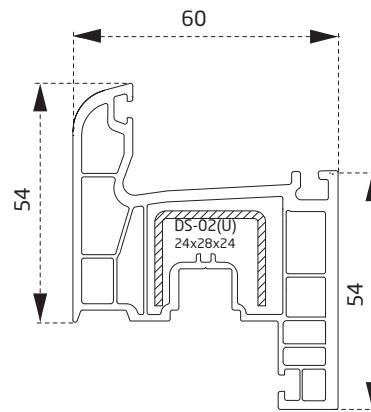
PRVNEC02B Kanat Profili Sash Profile
