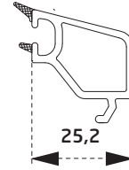
PDR1960BY 24 mm Cam Çıtası 24mm Glazing Bead
