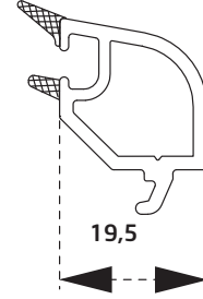
PVN1760BY 20 mm Cam Çıtası 20 mm Glazing Bead
