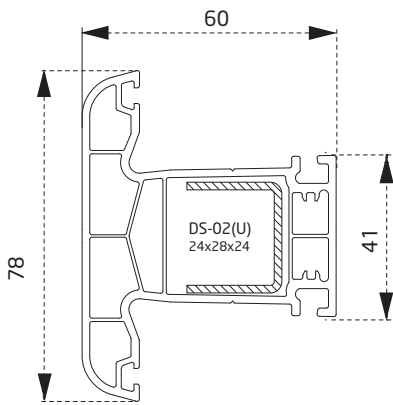
PRVNEC03B Orta Kayıt Profili Mullion Profile
