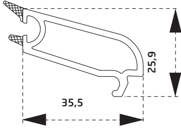
PVN1460BY Tek Cam Çıtası Single Glazing Bead
