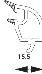
PVN1960BY 24 mm Cam Çıtası 24mm Glazing Bead
